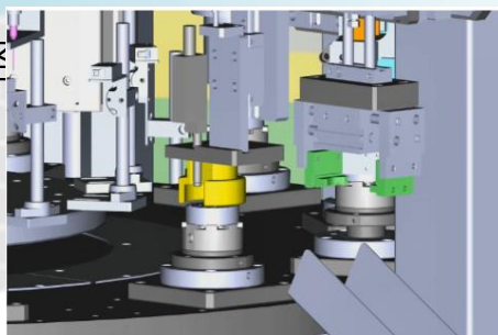
检测高度— 铁心高度量测(OK / NG)
