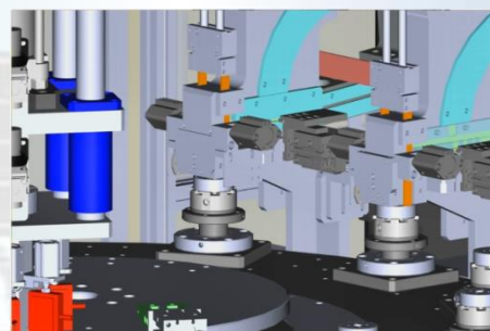
插入磁铁
